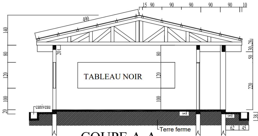
COUPE A-A
